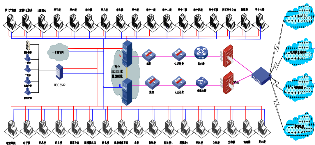
图 11-1 网络改造后网络拓扑图
